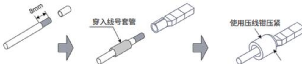
线缆制作图例
